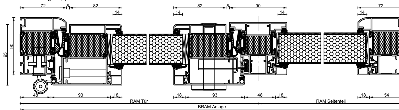
AluDesign 1-flgl. nach innen öffnend mit flächenversetztem Flügel Seitenteil als Pfostenkonstruktion
