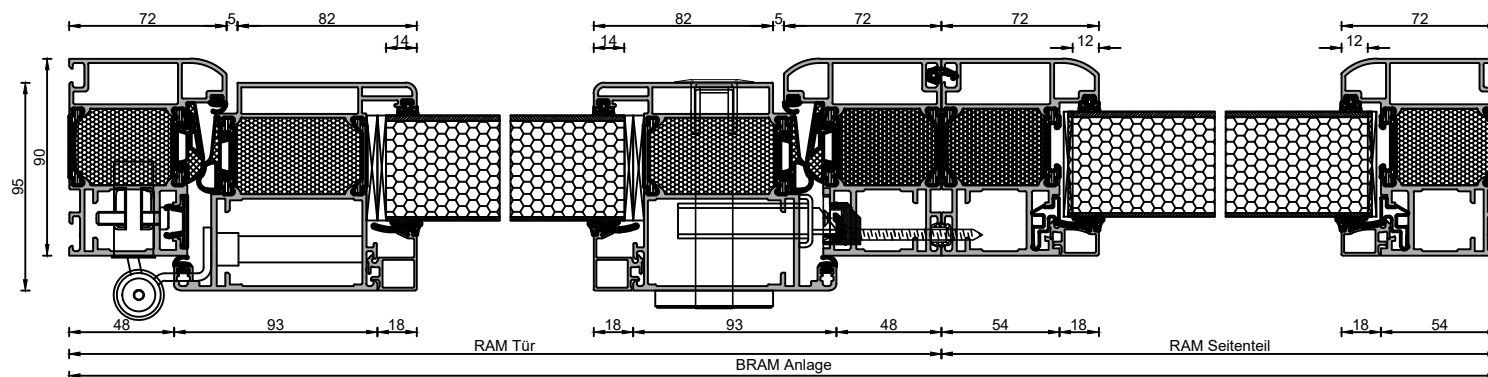
AluDesign 1-flgl. nach innen öffnend mit flächenversetztem Flügel Seitenteil gekoppelt
