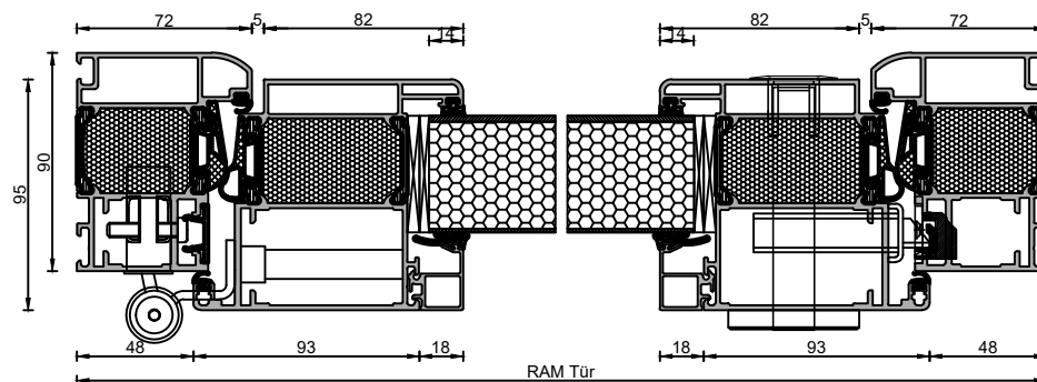
AluDesign 1-flgl. nach innen öffnend mit flächenversetztem Flügel
