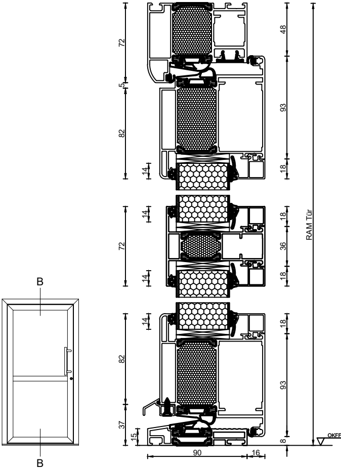
AluDesign 1-flgl. nach innen öffnend mit flächenversetztem Flügel Tür-Sprossenprofil glasteilend
