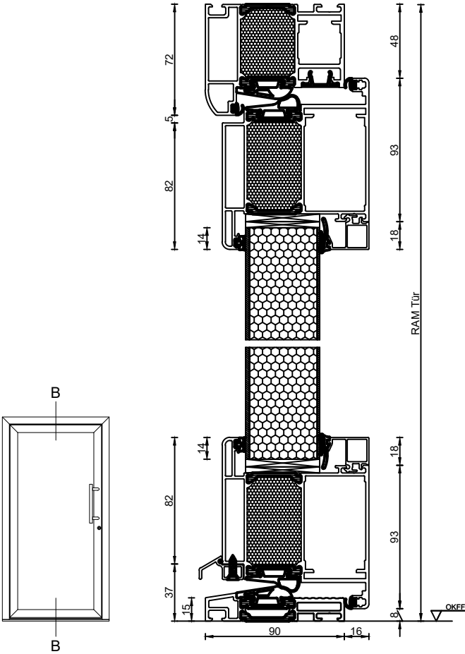
AluDesign 1-flgl. nach innen öffnend mit flächenversetztem Flügel
