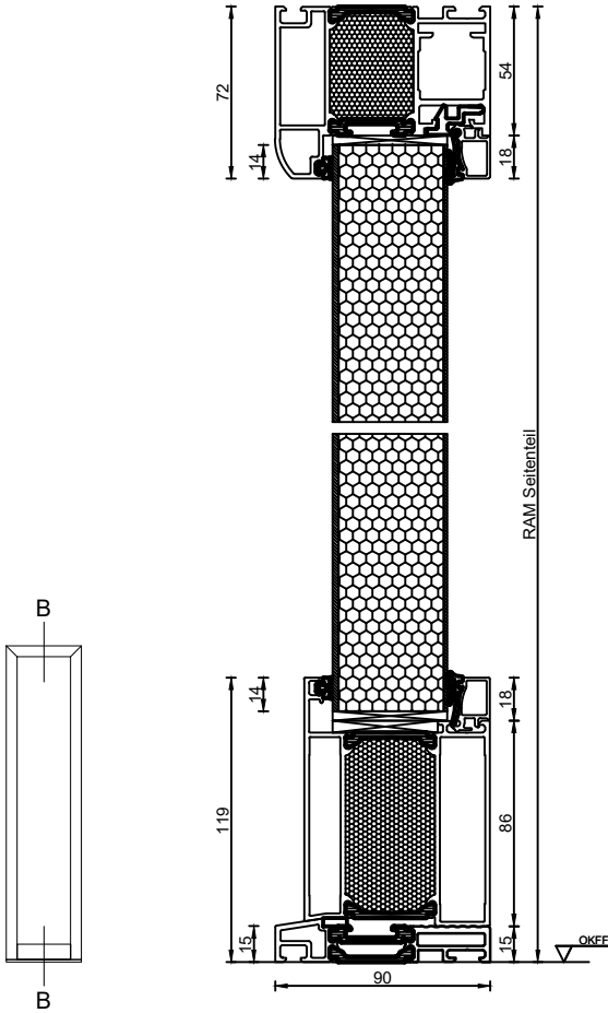
AluDesign Seitenteil
