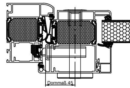
Glasfalzfüllung 34mm
