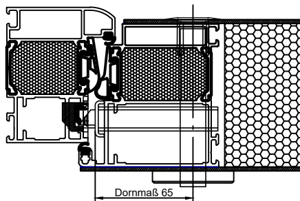
einseitig flügelüberdeckende Füllung
