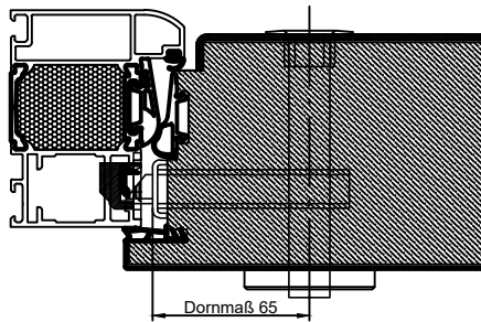
beidseitig flügelüberdeckende Füllung
