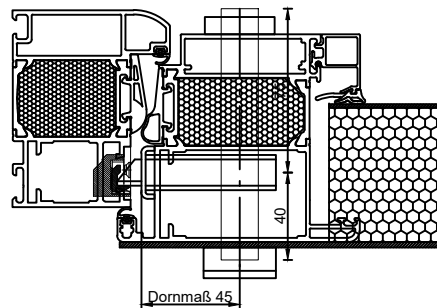
einseitig flügelüberdeckende Füllung
