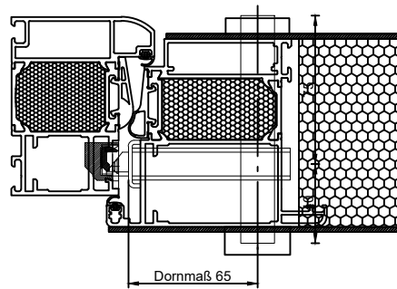
einseitig flügelüberdeckende Füllung
