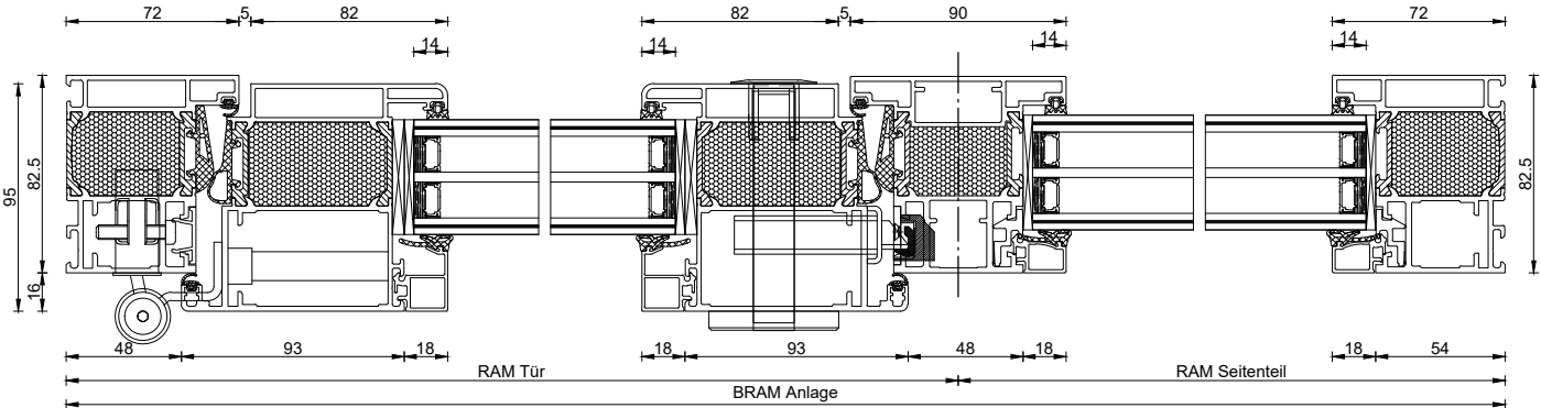
AluDesign 1-flgl. nach innen öffnend mit flächenversetztem Flügel Seitenteil als Pfostenkonstruktion
