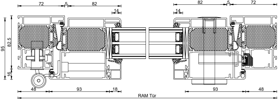
AluDesign 1-flgl. nach innen öffnend mit flächenversetztem Flügel
