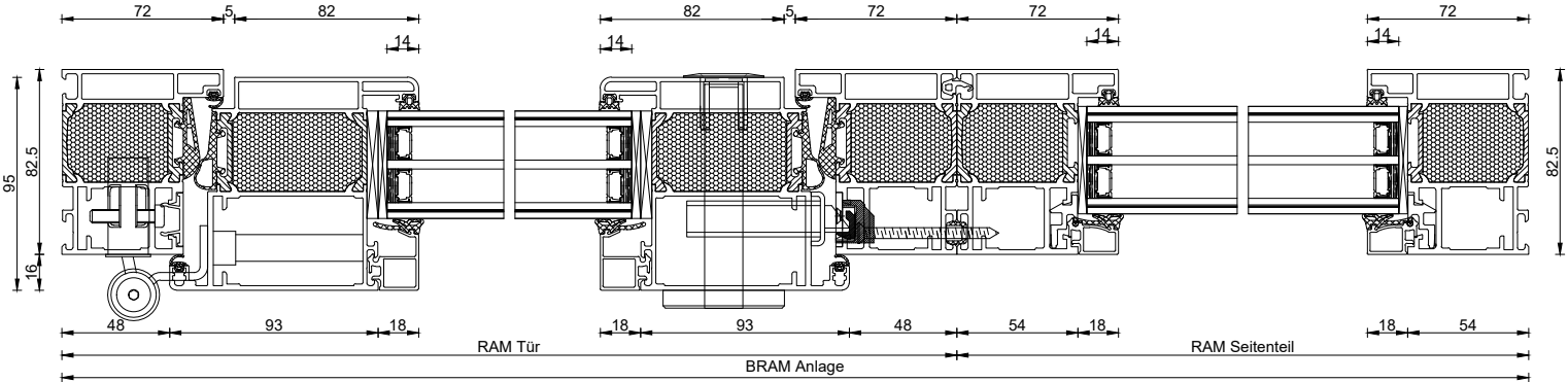
AluDesign 1-flgl. nach innen öffnend mit flächenversetztem Flügel Seitenteil gekoppelt
