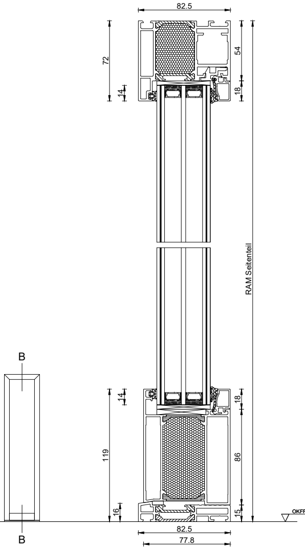
AluDesign Athos Seitenteil
