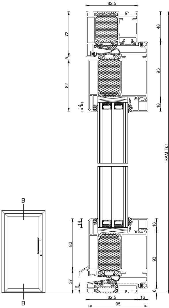
AluDesign Athos 1-flg. nach innen öffnend mit flächenversetztem Flügel
