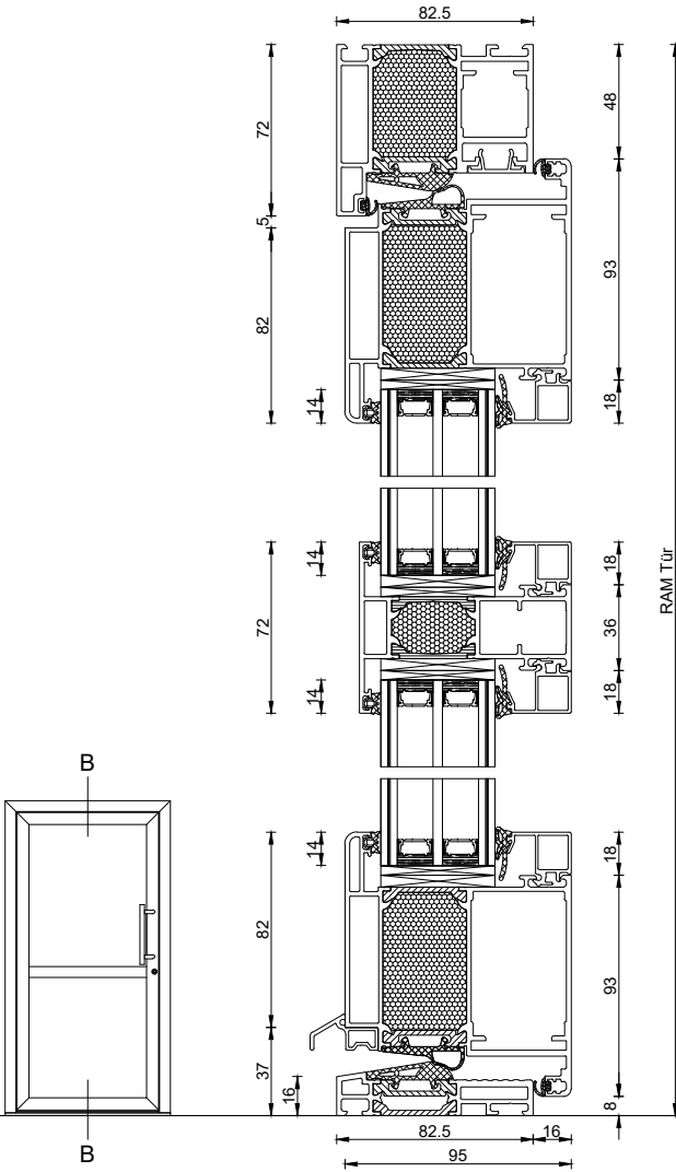
AluDesign Athos 1-flg. nach innen öffnend mit flächenversetztem Flügel
