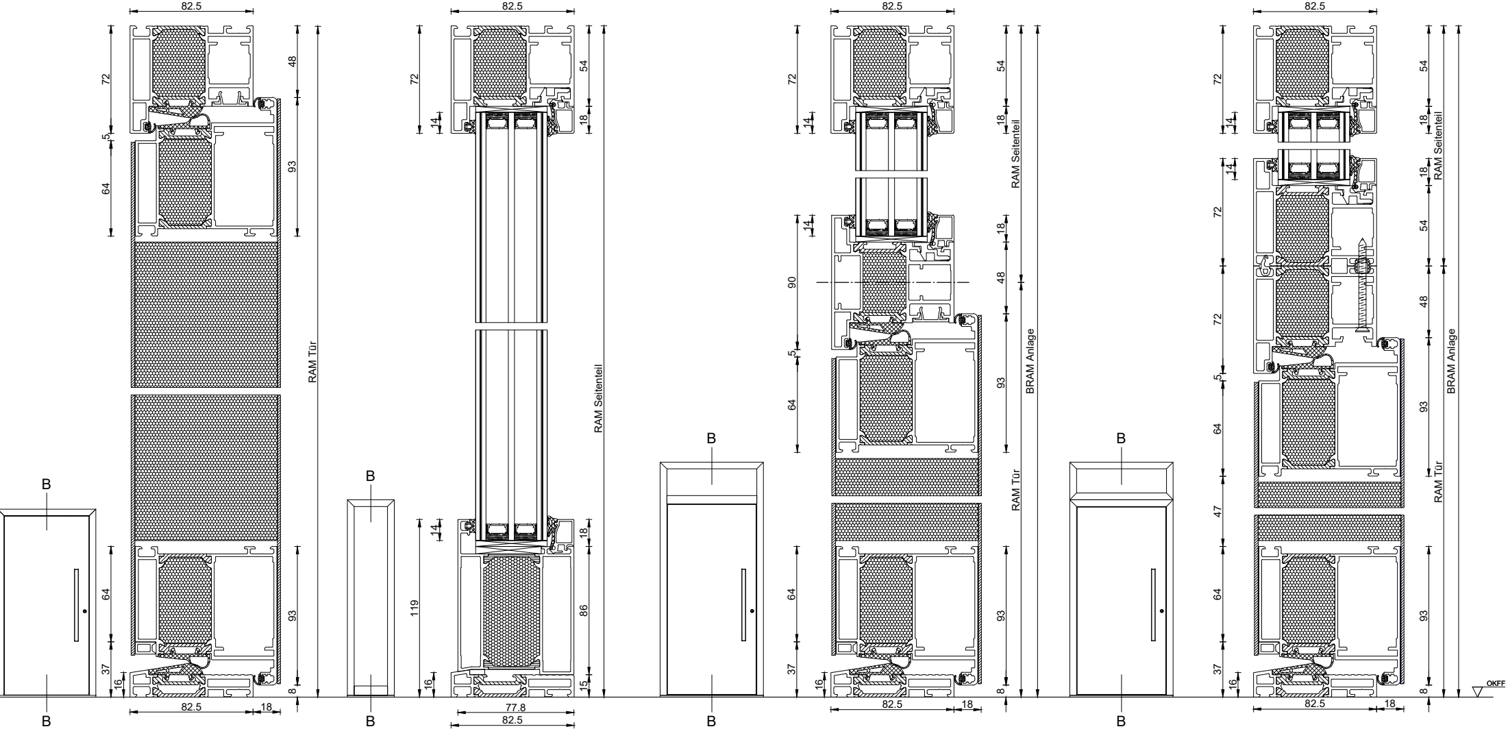
AluDesign 1-flgl. nach innen öffnend mit flächenversetztem Flügel
