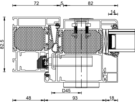
Glasfalzfüllung 34mm
