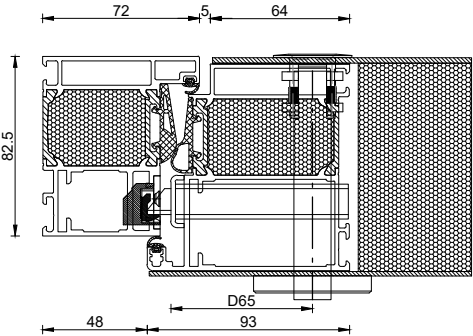
beidseitig flügelüberdeckende Füllung
