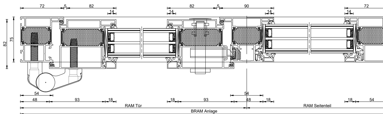
AluDesign Porthos 1-flg. nach innen öffnend Seitenteil als Pfostenkonstruktion
