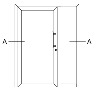
AluDesign Porthos 1-flg. nach innen öffnend Seitenteil als Pfostenkonstruktion
