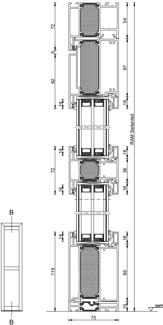
AluDesign Porthos Seitenteil Ausgleichsprofil, Seitenteil-Sprossenprofil glasteilend
