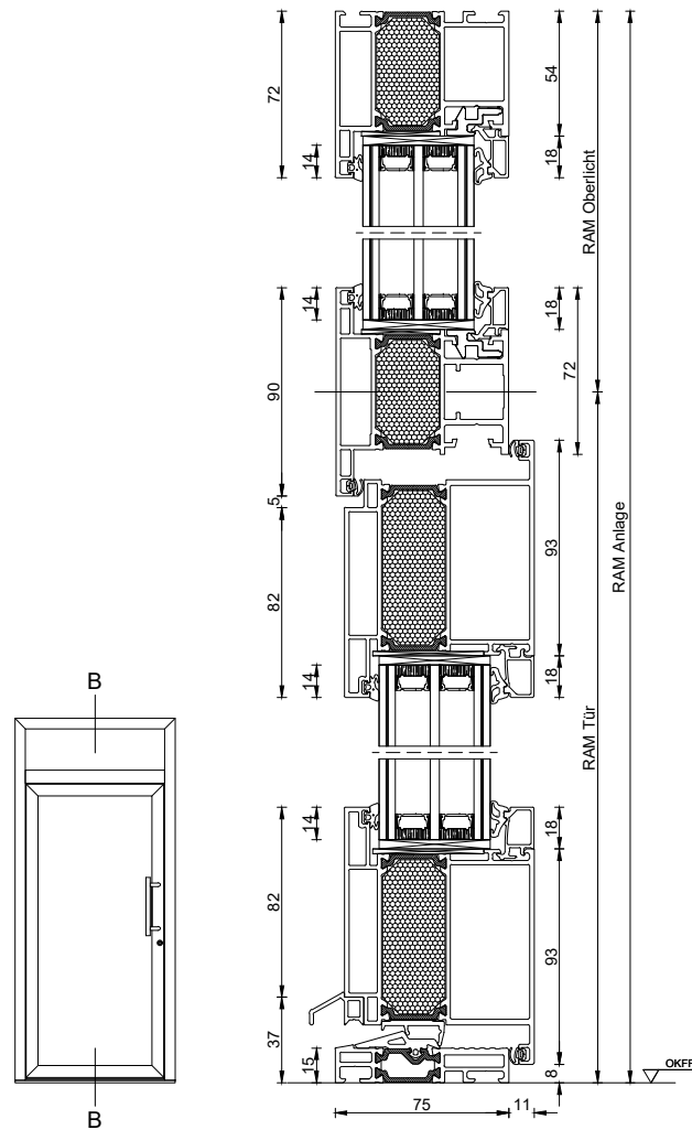
AluDesign Porthos 1-flgl. nach innen öffnend Oberlicht als Pfostenkonstruktion
