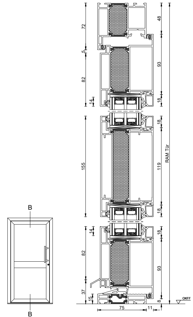
AluDesign Porthos 1-flgl. nach innen öffnend Quersfries glasteilend
