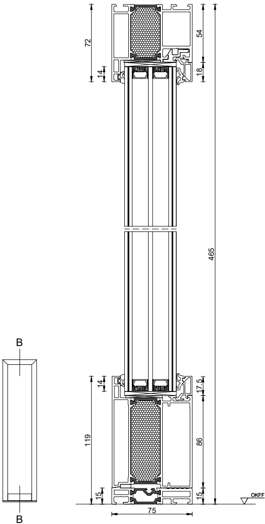
AluDesign Porthos Seitenteil
