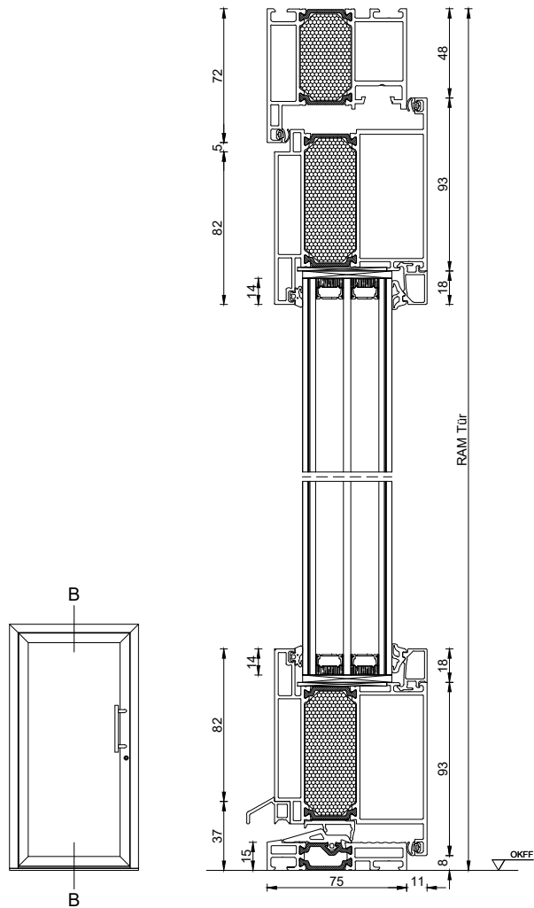
AluDesign Porthos 1-flgl. nach innen öffnend
