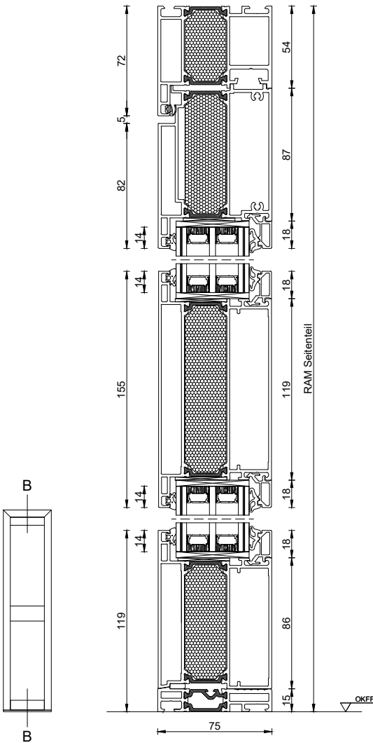
AluDesign Porthos Seitenteil Ausgleichsprofil, Querfries glasteilend
