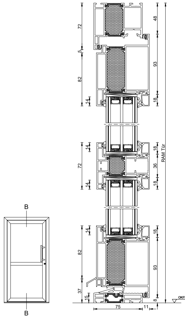
AluDesign Porthos 1-flgl. nach innen öffnend Tür-Sprossenprofil glasteilend
