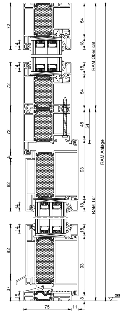
AluDesign Porthos 1-flgl. nach innen öffnend Oberlicht gekoppelt
