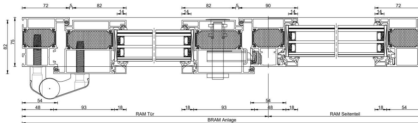
AluDesign Porthos 1-flgl. nach innen öffnend Seitenteil als Pfostenkonstruktion
