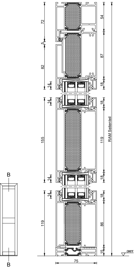
AluDesign Porthos Seitenteil Ausgleichsprofil, Querrfries glasteilend
