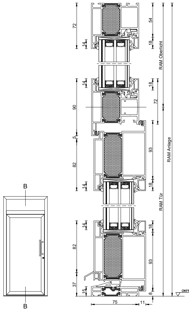
AluDesign Porthos 1-flg. nach innen öffnend Oberlicht als Pfostenkonstruktion
