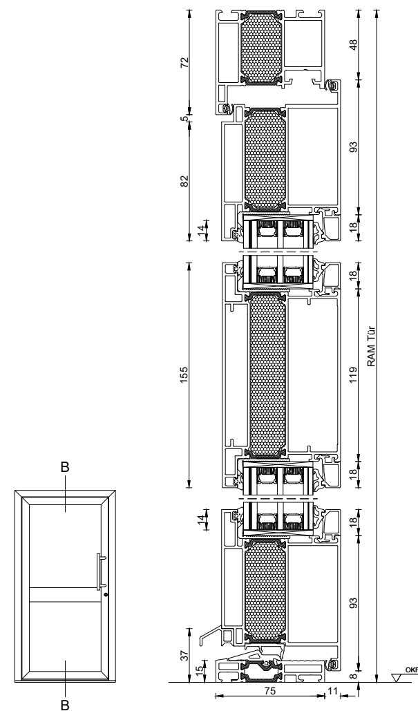
AluDesign Porthos 1-flgl. nach innen öffnend Querfries glasteilend
