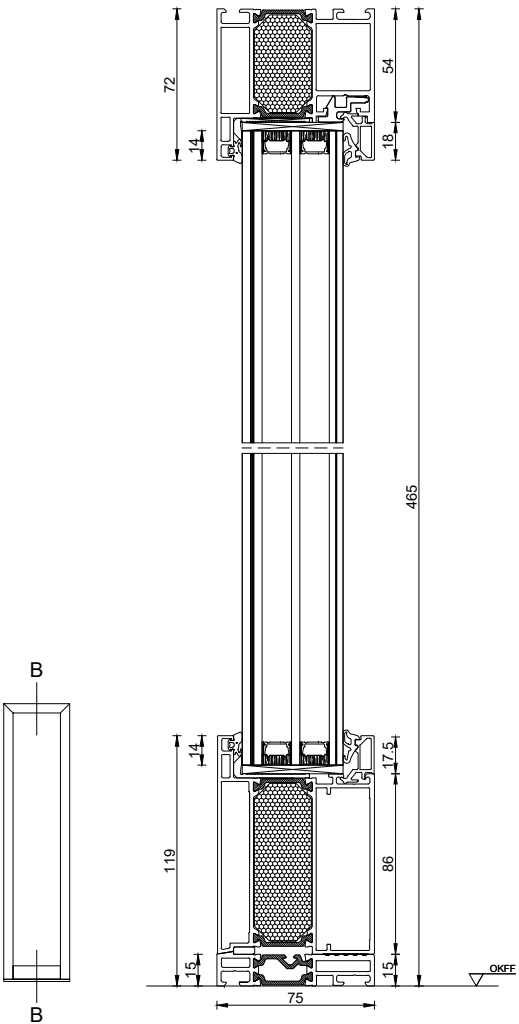
AluDesign Porthos Seitenteil
