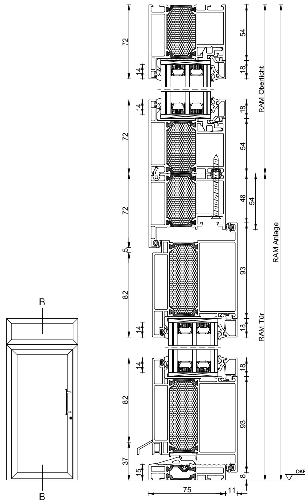
AluDesign Porthos 1-flg. nach innen öffnend Oberlicht gekoppelt
