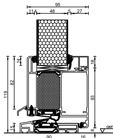
Bodenanschluss Türflügel Ausführung Glasfalzfüllung 48 mm
