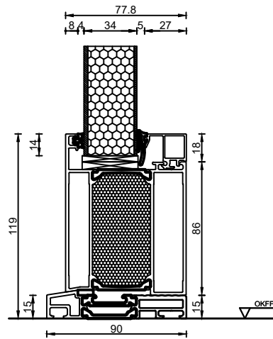
Bodenanschluss Sockelprofil auf Schwelle im Seitenteil Ausführung Glasfalzfüllung 34 mm
