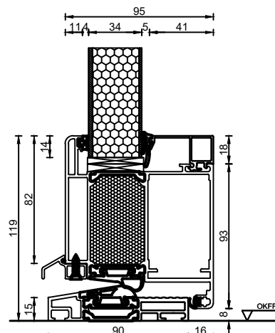
Bodenanschluss Türflügel Ausführung Glasfalzfüllung 34 mm
