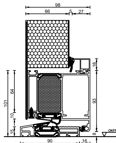
Bodenanschluss Türflügel Ausführungs-Paket 1 einseitig flügelüberdeckend 66 mm
