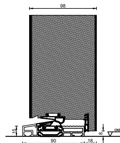
Bodenanschluss Türflügel Ausführungs-Paket 3 Vollblatt-Flügel 98 mm
