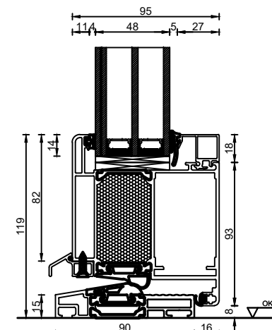
Bodenanschluss Türflügel Ausführung Isolierverglasung 48 mm
