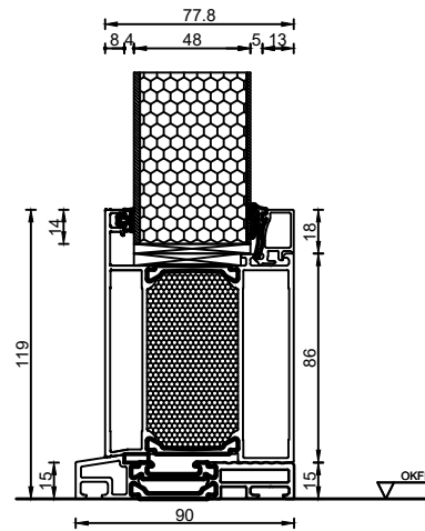
Bodenanschluss Sockelprofil auf Schwelle im Seitenteil Ausführung Glasfalzfüllung 48 mm
