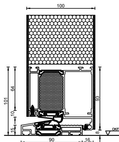
Bodenanschluss Türflügel Ausführungs-Paket 2 beidseitig flügelüberdeckend 100 mm
