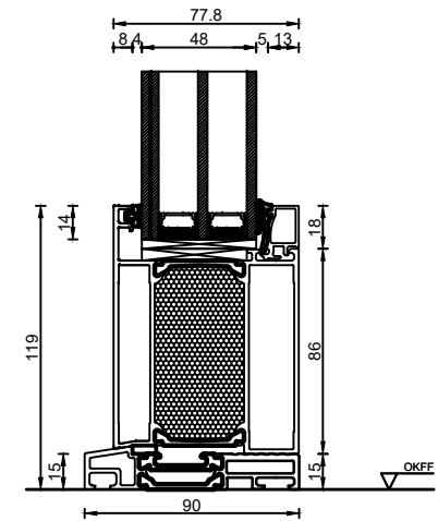
Bodenanschluss Sockelprofil auf Schwelle im Seitenteil Ausführung Isolierverglasung 48 mm
