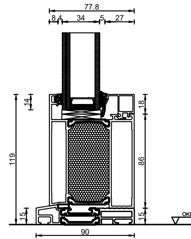
Bodenanschluss Sockelprofil auf Schwelle im Seitenteil Ausführung Isolierverglasung 34 mm
