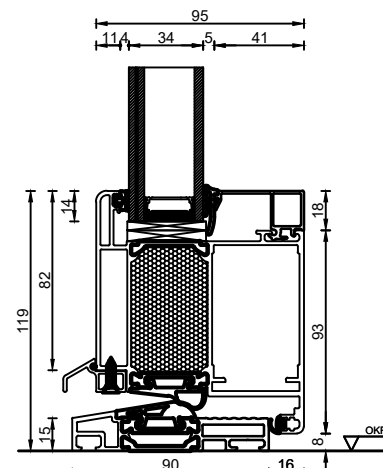
Bodenanschluss Türflügel Ausführung Isolierverglasung 34 mm
