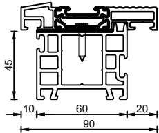
Bodenschwelle Unterbauprofil konstruktiv durchlaufend unter der Schwelle in Tür und Seitenteil
