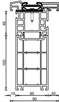
Pfosten mit Stabilisierungsprofil
