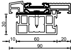
Bodenschwelle Unterbauprofil konstruktiv durchlaufend unter der Schwelle in Tür und Seitenteil
