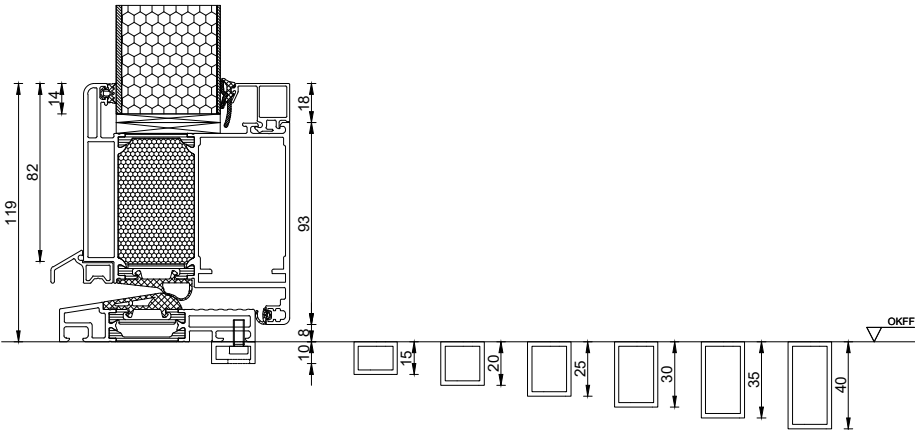
Bodenschwellenunterbau Aluminium-Rechteckrohr auf der Innen oder Außenseite an Tür und Seitenteil
