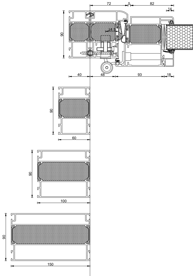
Zusatzprofile seitlich und oben an Tür und Seitenteil / Oberlicht
