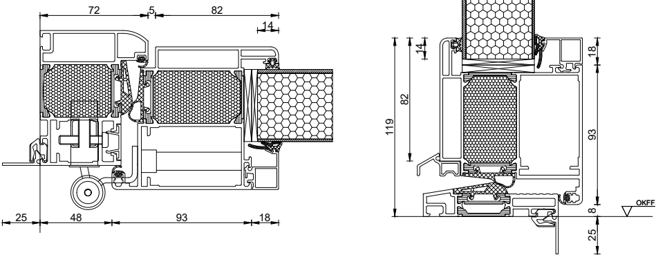
Wandanschlussprofile seitlich, oben und unter der Schwelle an Tür und Seitenteil / Oberlicht
