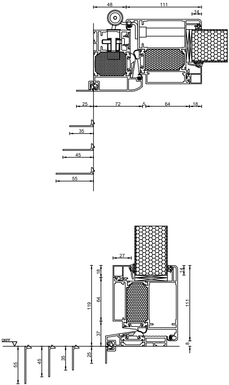
Wandanschlussprofile seitlich, oben und unter der Schwelle an Tür und Seitenteil / Oberlicht
