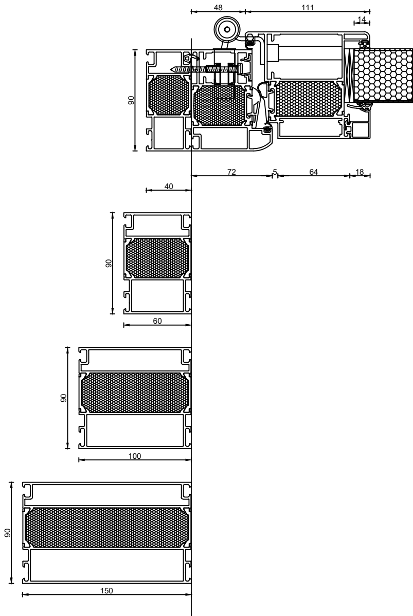
Zusatzprofile seitlich und oben an Tür und Seitenteil / Oberlicht
