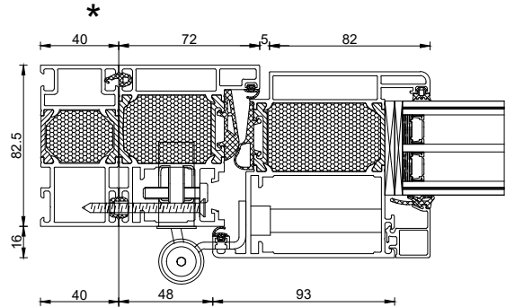
Zusatzprofile seitlich und oben an Tür und Seitenteil / Oberlicht
