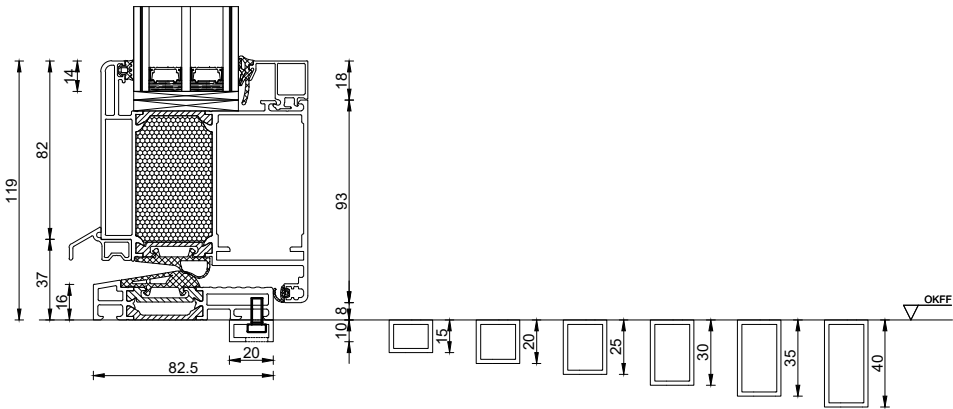
Bodenschwellenunterbau Aluminium-Rechteckrohr auf der Innen oder Außenseite an Tür und Seitenteil
