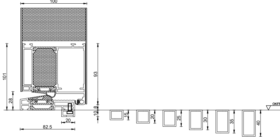
Bodenschwellenunterbau Aluminium-Rechteckrohr auf der Innen oder Außenseite an Tür und Seitenteil
