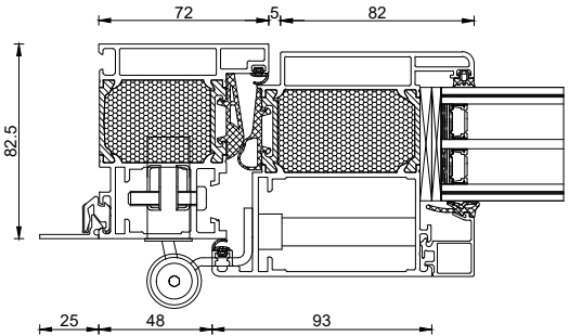
Wandanschlussprofile seitlich, oben und unter der Schwelle an Tür und Seitenteil / Oberlicht
