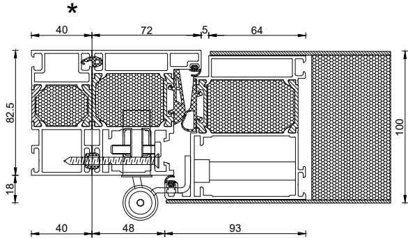
Zusatzprofile seitlich und oben an Tür und Seitenteil / Oberlicht
