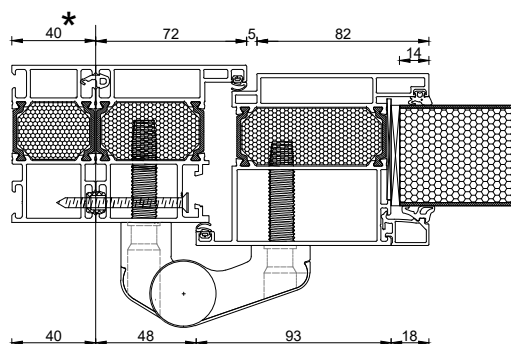
Zusatzprofile seitlich und oben an Tür und Seitenteil / Oberlicht
