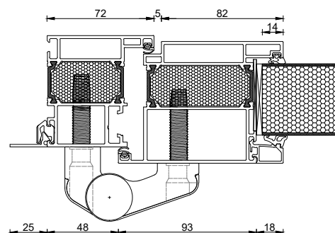
Wandanschlussprofile seitlich, oben und unter der Schwelle an Tür und Seitenteil / Oberlicht
